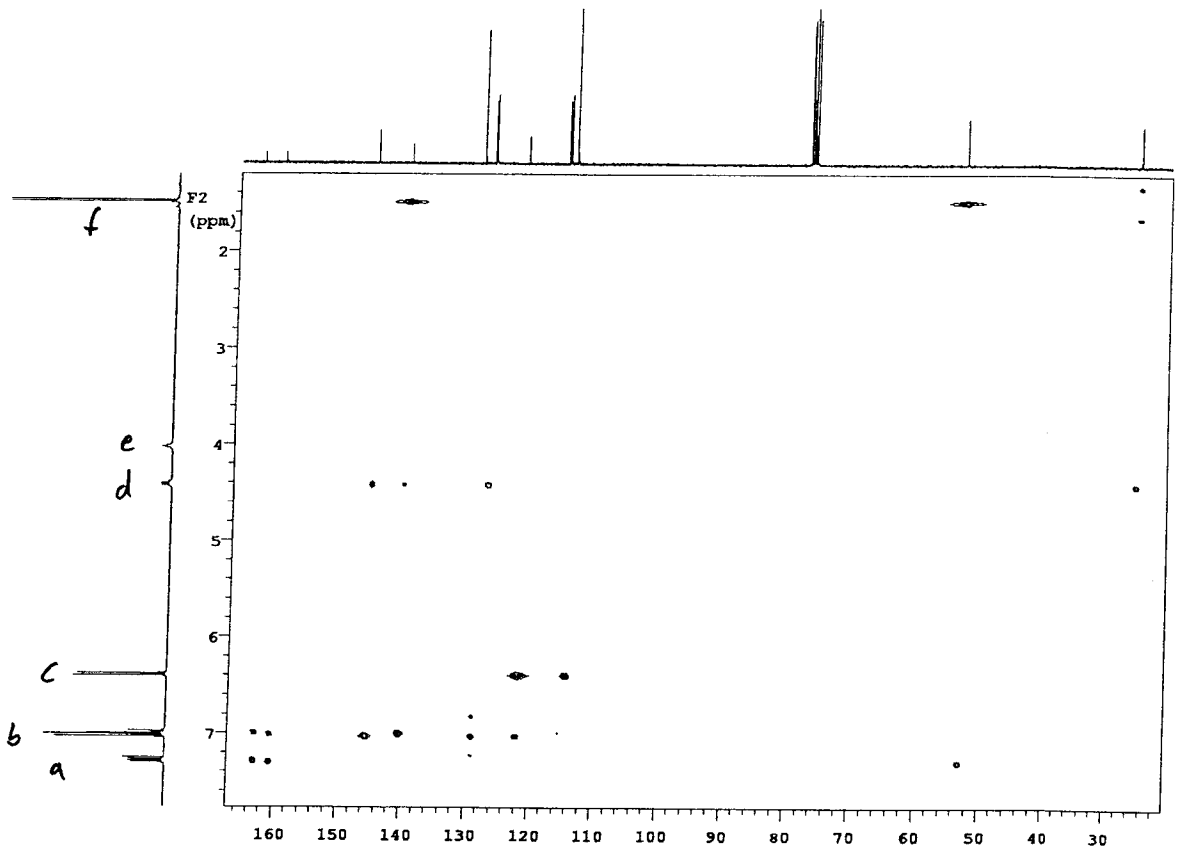
HMBC
