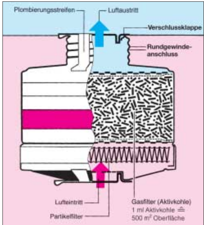
Bild 23: Kombinationsfilter
