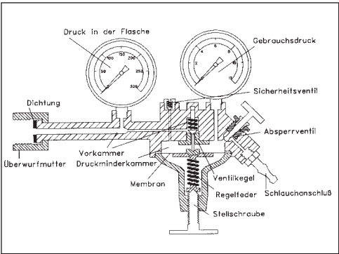
Schema eines Druckminderers
